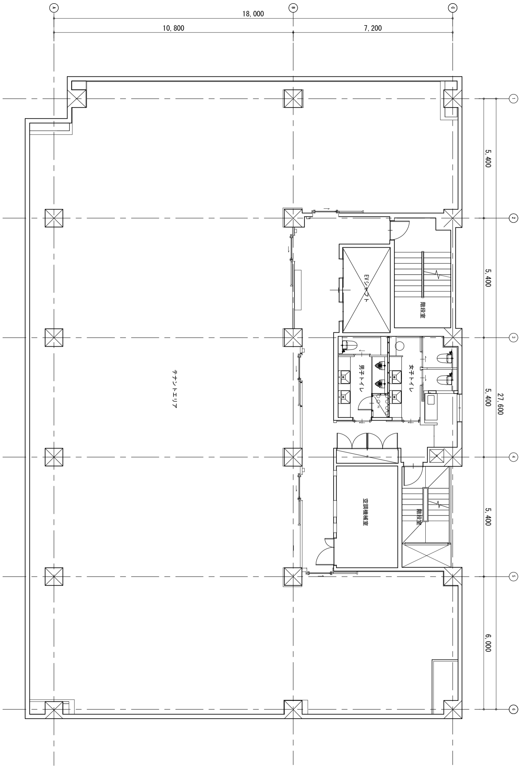
7～9階平面図
